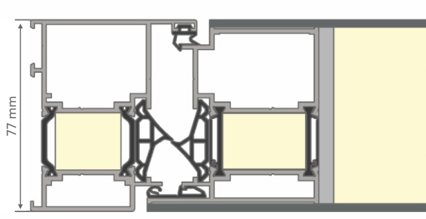
DRZWI Z PANELEM 2-STRONNIE LICOWANYM WERSJA Z USZCZELKĄ CENTRALNĄ
